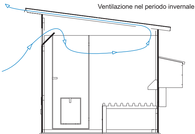
Schema dei flussi di ventilazione naturale del tipo "a camino".
